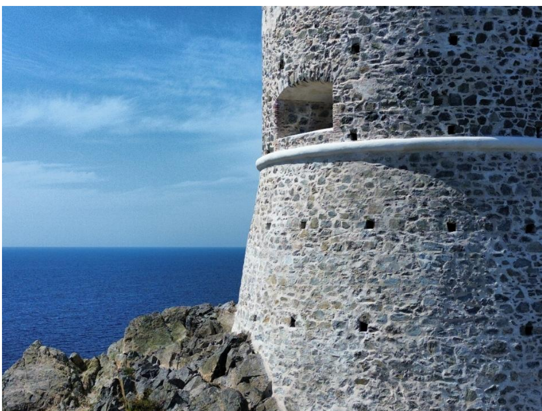
Détails de la reprise du cordon intermédiaire en brique puis enduit
